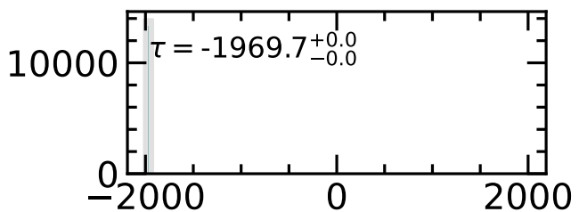
PyROA
