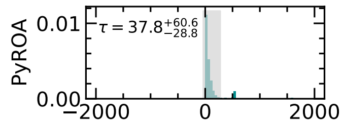
Lag [days]
