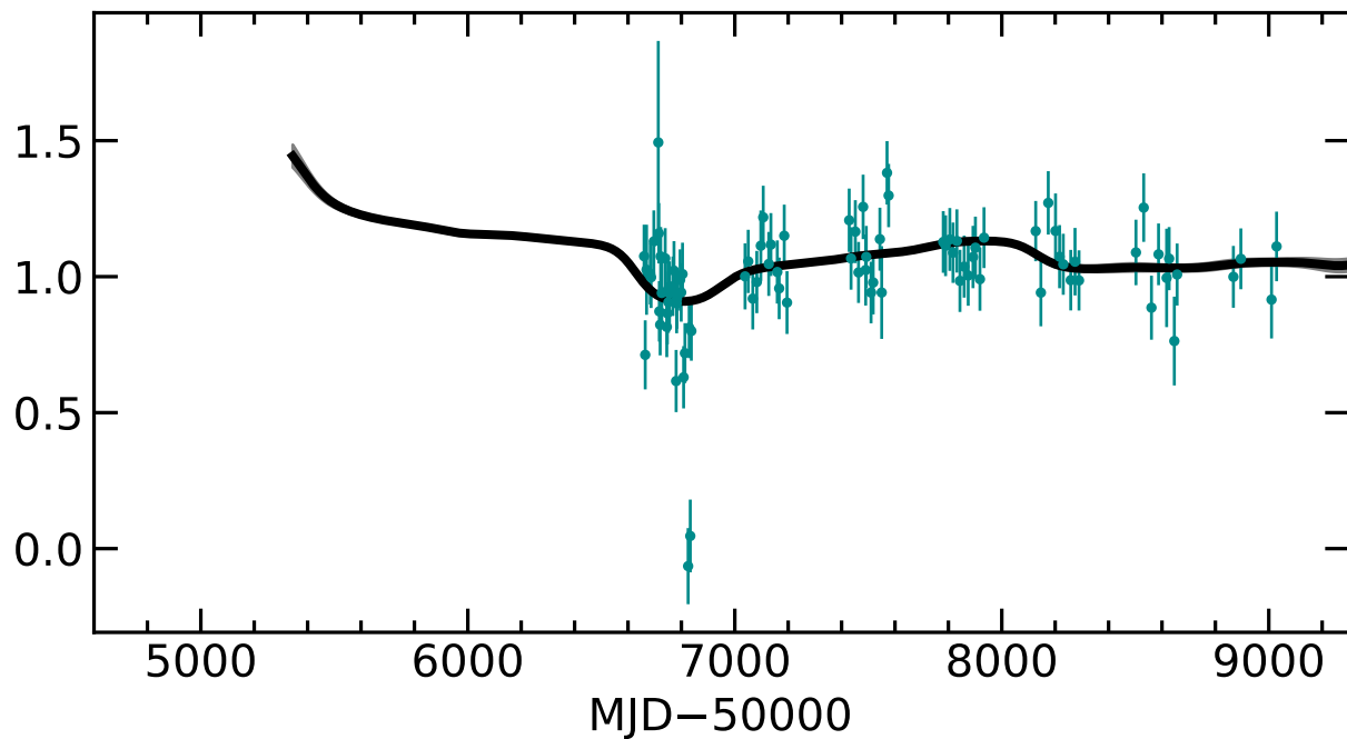
PyROA
