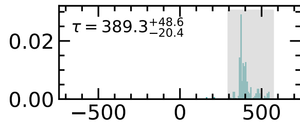
CCCD
