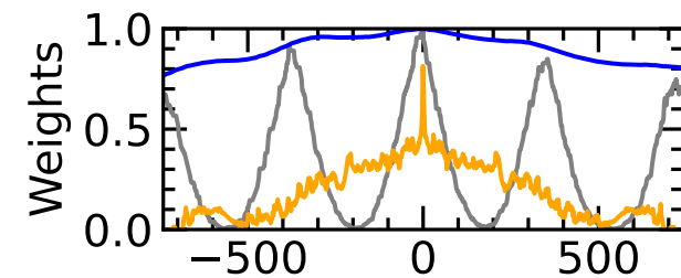
CCCD
