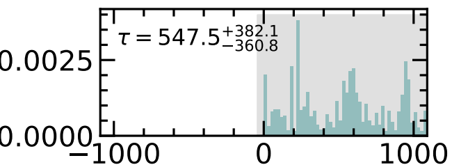
PyROA
