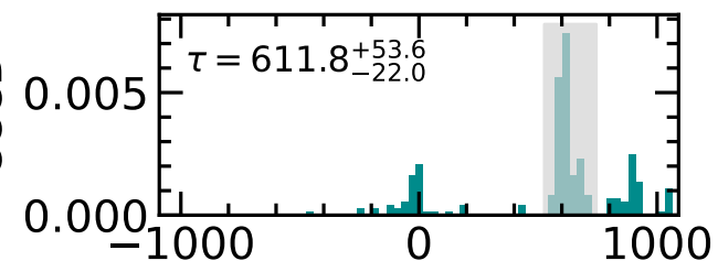
CCCD
